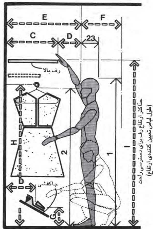
کمد و محفظه‌ی لباس، زنانه
