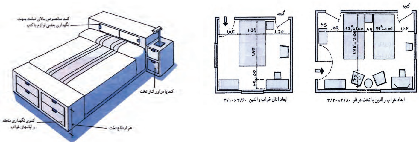
تصویر ۳-۴۶- ابعاد و مبلمان نمونه‌هایی از اتاق خواب والدین
