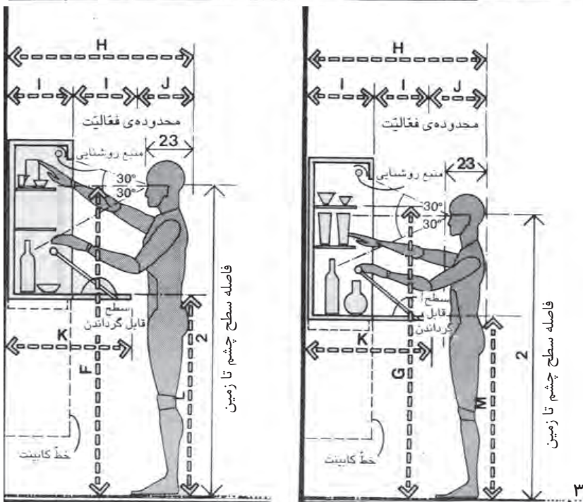
ویرترین نصب شده بر دیوار، دسترسی فرد مؤنث و ویرترین نصب شده بر دیوار، دسترسی فرد مذکر
