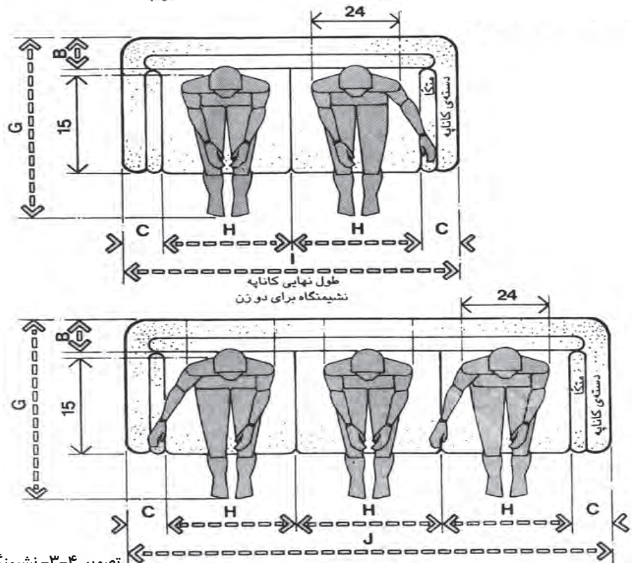
تصویر ۳-۴- نشیمنگاه کاناپه‌ای افراد مؤنث (اندازه درج شده بر روی ترسیمات به اینچ می‌باشد).
