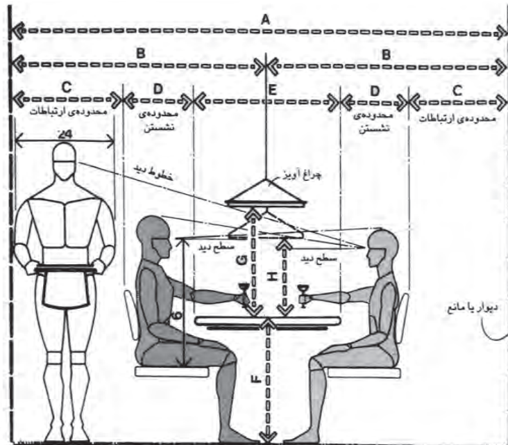
تصویر ۱۷-۳- حداقل پهنای محدوده‌ی غذایی
